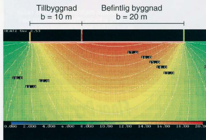
Figur 7: Förväntade temperaturnivåer under betongplattorna efter tillbyggnad. 200 mm värmeisolering under tillbyggd platta.
