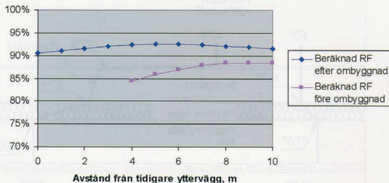
Figur 8: RF i befintlig byggnad före respektive efter tillbyggnad.
