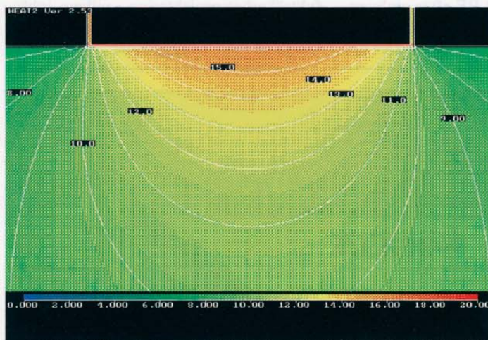
Figur 4: Förväntade temperaturnivåer under betongplatta på mark med bredden 20 m och underliggande värmeisolering i form av 80 mm XPS-isolering. \lambda_{\text{mark}} = 2,0 \text{ W/mK} , motsvarar sand/morän,
