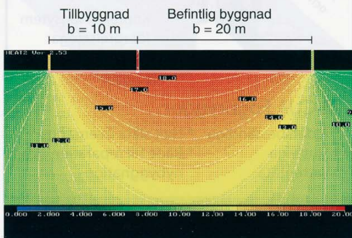
Figur 6: Förväntade temperaturnivåer under betongplattorna efter tillbyggnad. 100 mm värmeisolering under tillbyggd platta.
