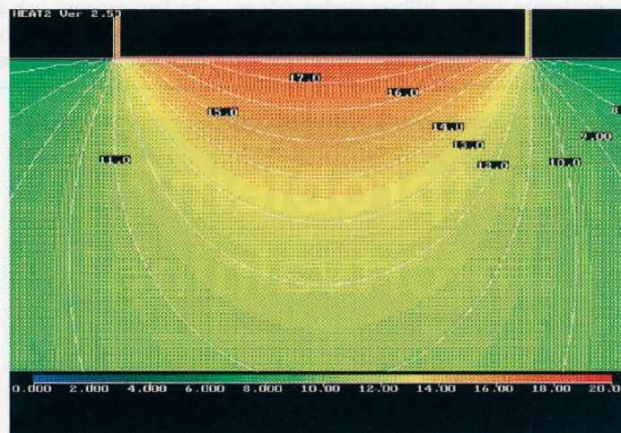
Figur 5: Förväntade temperaturnivåer under betongplatta på mark med bredden 20 m och underliggande värmeisolering i form av 80 mm XPS-isolering. \lambda_{\text{mark}} = 1,0 \text{ W/mK} , motsvarar lera.
